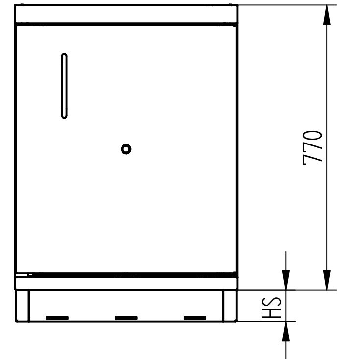
ToeKick-Sockel
