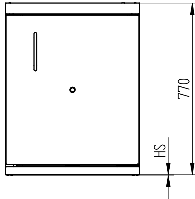
Außenboden
